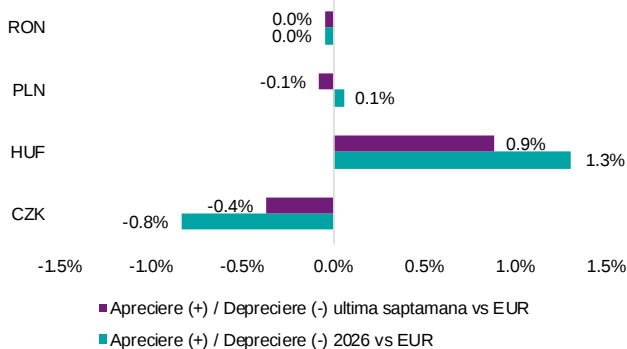
Evoluția monedelor din Europa Centrală și de Est față de euro
