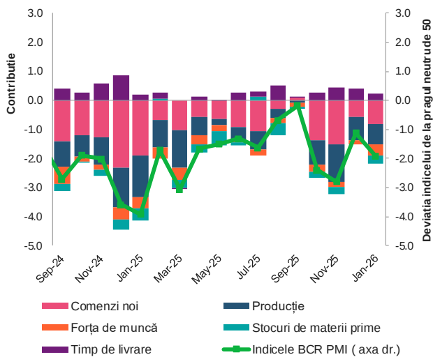
Evoluția BCR PMI privind industria prelucrătoare din România
