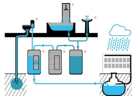
Schéma využití šedé vody
