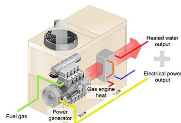
Schéma kogenerační jednotky (výroba tepla a elektrické energie)
